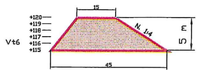
Tyyppipolkkleikkaus 1:1000/ 1:400
